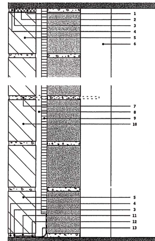
Fassadendetail Kopf- und Fusspunkt
